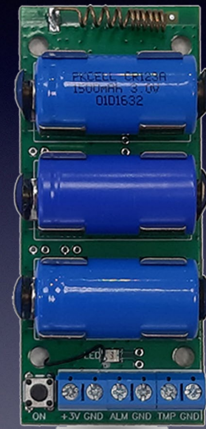
U-Prox WirePort
